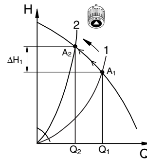
Obr. 11 Neregulované čerpadlo
